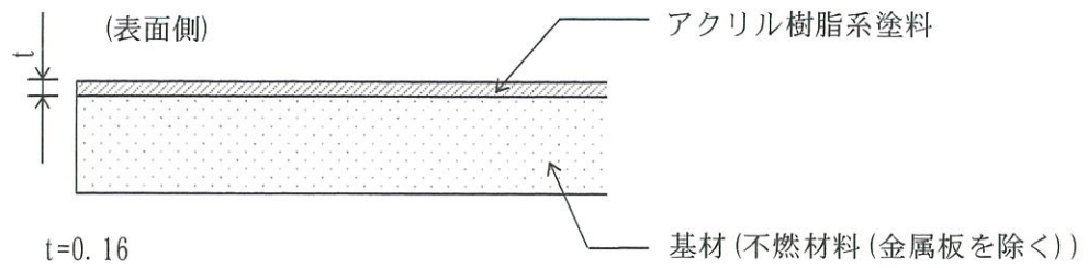
図 1 断面図
