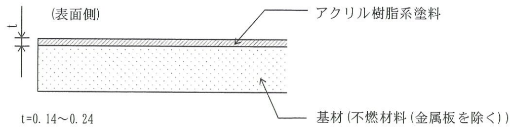
図 1 断面図
